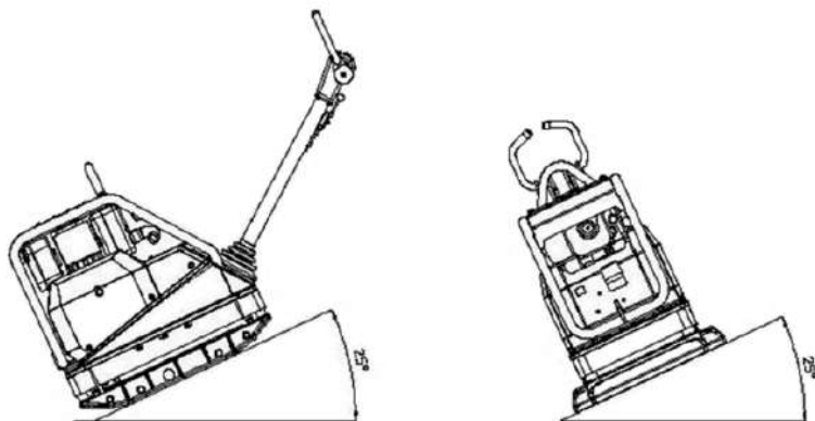
Рис. 2. Допустимый наклон виброплиты
